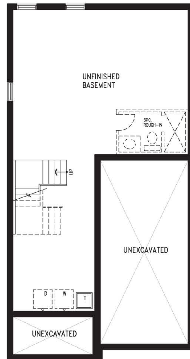
BASEMENT PLAN 'A' & 'B'
