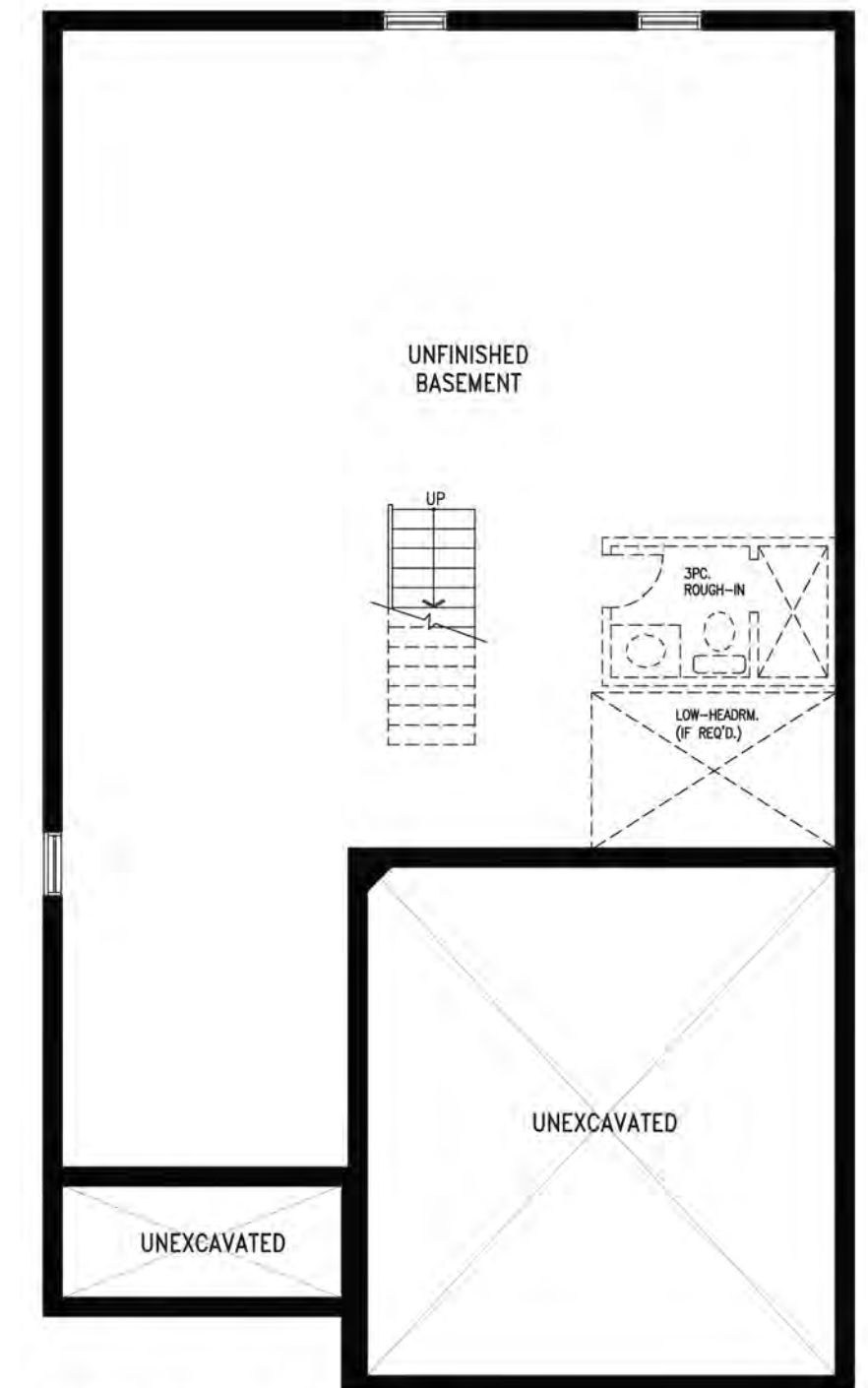
BASEMENT PLAN 'A' & 'B'
