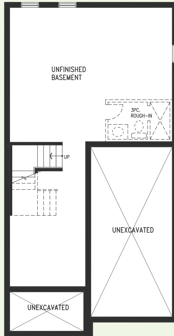
BASEMENT PLAN 'A' & 'B'
